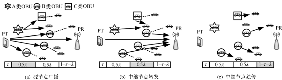
图 2 单小区认知协作频谱共享模型
